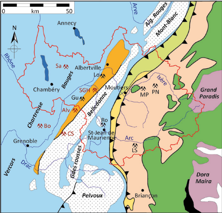
Carte géologique simplifiée de la Savoie avec localisation des principales mines. Alv: Alleverd, Bo: Bovinant, CS: mine de fer, col de Sitre, Gu: Guerraz, Lo: Longera, LS: Les Sarrasins, MP: Mâcot-La Plagne, PN: Peisey-Nancroix, Ro: Rocheray, Sa: Sambuy + Semnoz, SGH: mine des Hurtières.
