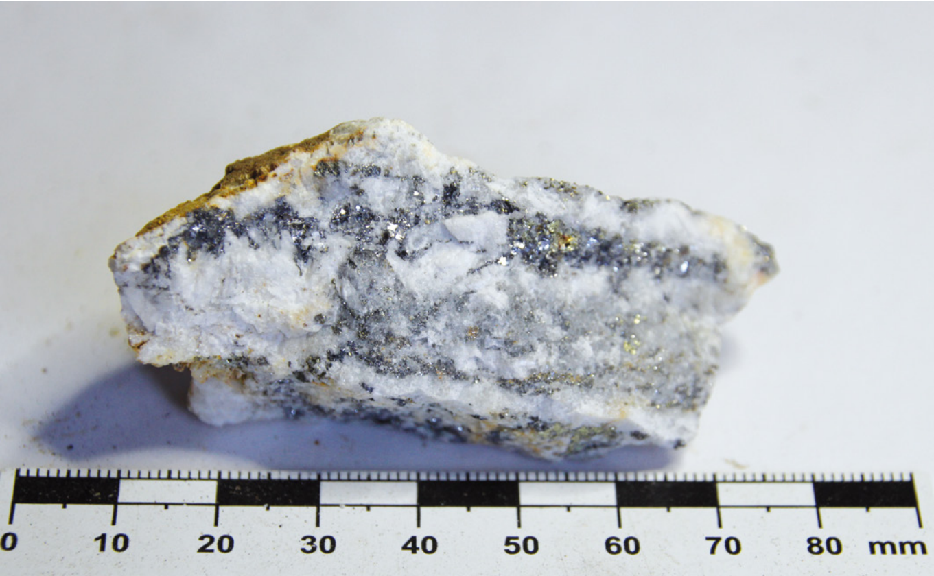
Minerai de Pb-Zn-Ag (mine du Longeray) : galène argentée, chalcopryrite dorée et tétraédrite brune, dans une gangue de quartz.
