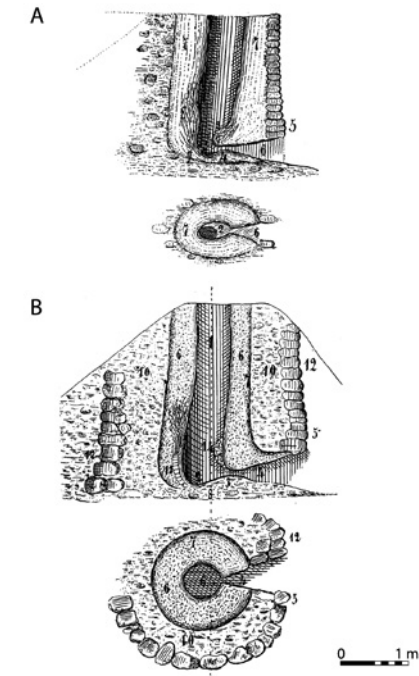
Esquisse du type de fourneau à ventilation naturelle relevé par Auguste Quiquerez dans le Jura suisse au XIX e siècle et identifié en fouilles sur le Salève pendant les campagnes conduites en 2013-2015 par Sébastien Perret. D'après Quiquerez 1992 [1866].
